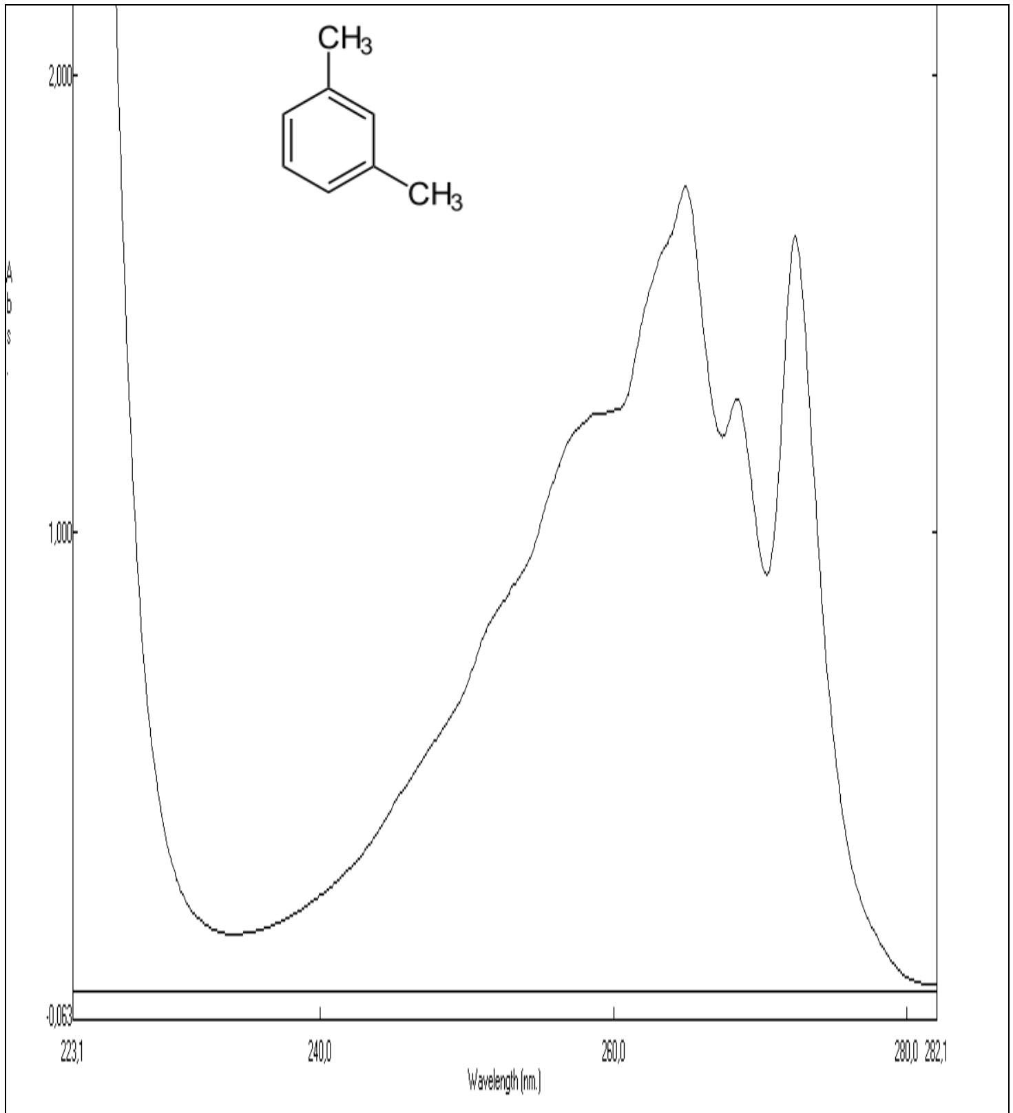
m-ξυλόλιο
