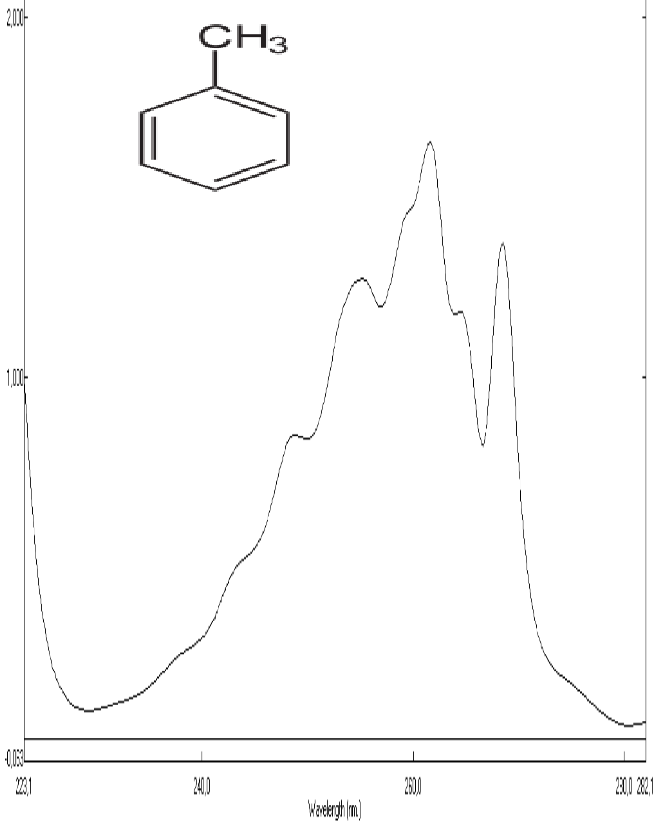
Τολουόλιο
